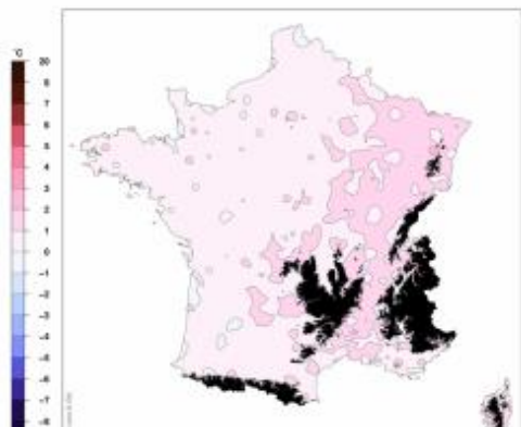
Température moyenne : été 2012 Ecart à la moyenne de référence 1981-2010
