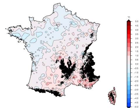
Température moyenne : été 2012 Ecart à la moyenne de référence 1981-2010
