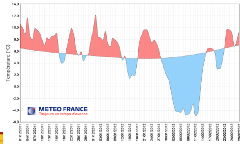
Evolution de la température en France au cours de l'hiver 2011-2012
